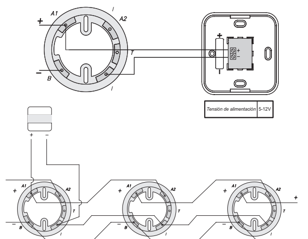
Esquema de conexionado sistema convencional
